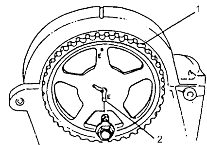
1. 凸轮轴正时皮带轮 2. 止推销
