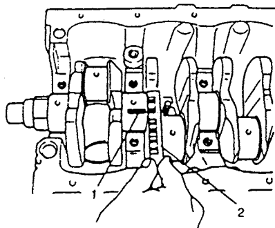
1. 塑料塞规 2. 比例尺
